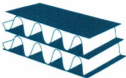
cartón corrugado doble
